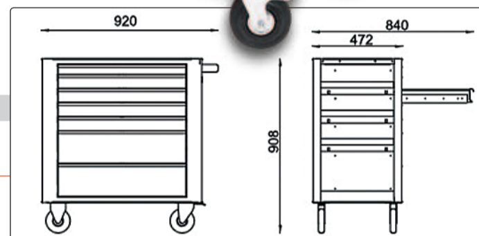
Размеры тележек CIMCO. Максимальная грузоподъемность 280 кг. Собственный вес 74 кг.
